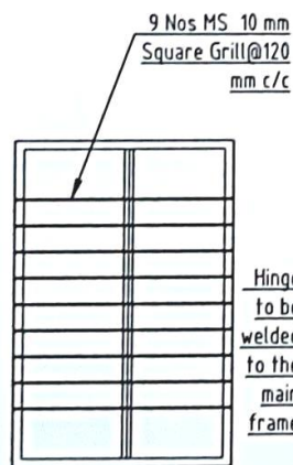
Window 2 : 1000 x 1500
